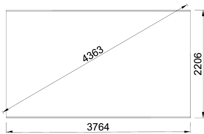
Sockelmaß Luna 2
